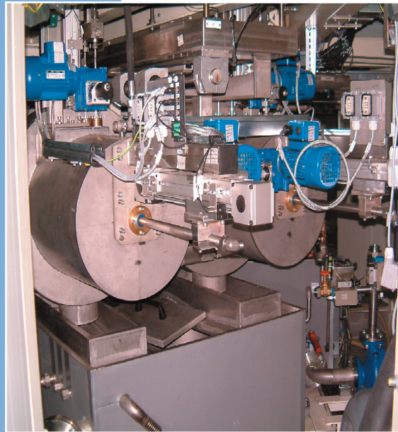
Behandlungskammern der MTM-Anlage Typ SKR 6HD-VAC
