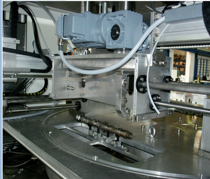
Werkstück an der Spülstation
