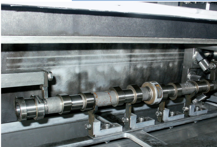
Strahldüsen (rechts außen) beim Entgraten
